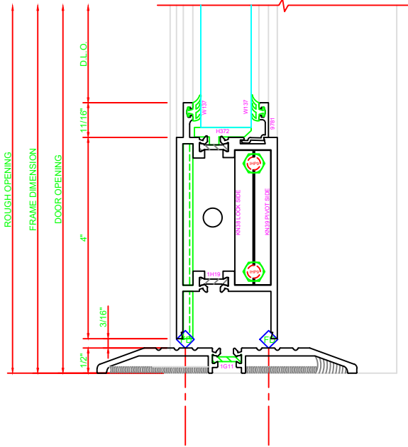
200 BOTTOM RAIL S/A D202
